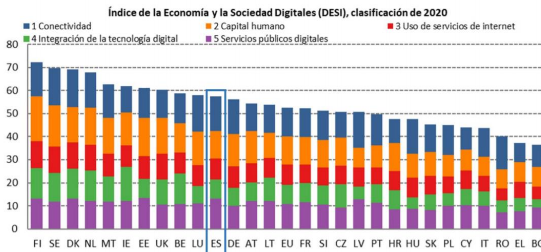
Figura 2 DESI 2020
